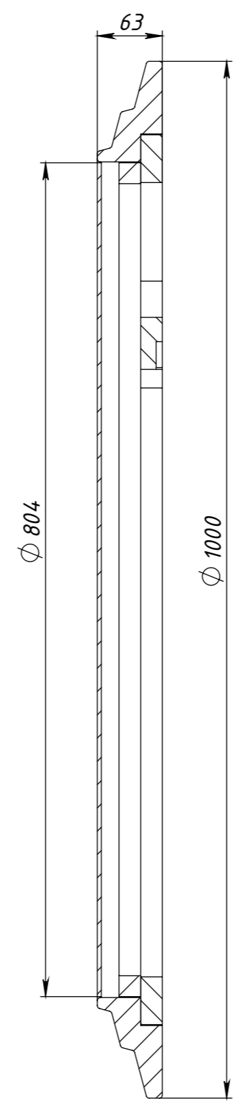
СЕЧЕНИЕ А-А МАСШТАБ 1 : 5
