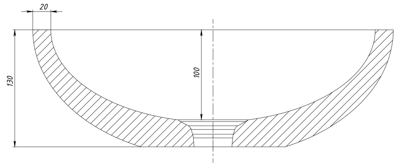
СЕЧЕНИЕ А-А МАСШТАБ 1 : 2
